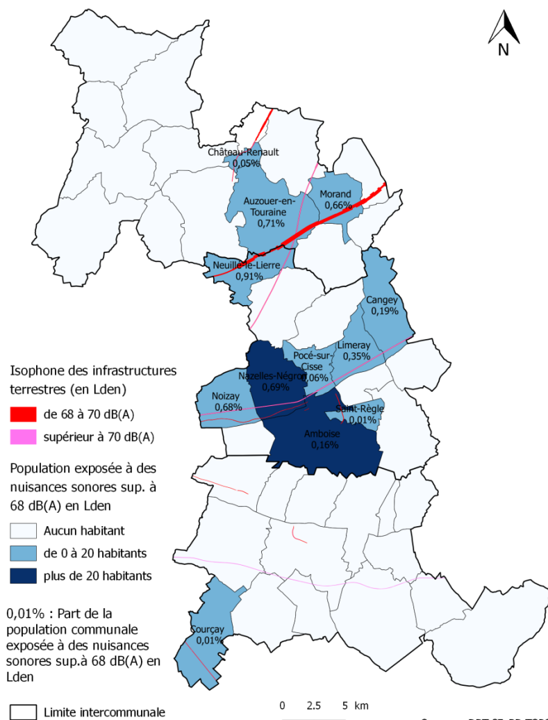
Estimation de la population exposée à des nuisances sonores supérieures à 68 dB(A) en Lden sur le territoire du SCoT ABC
